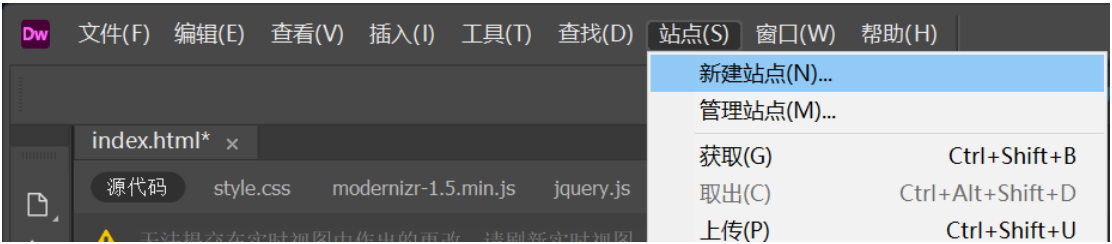
图 3 新建站点
