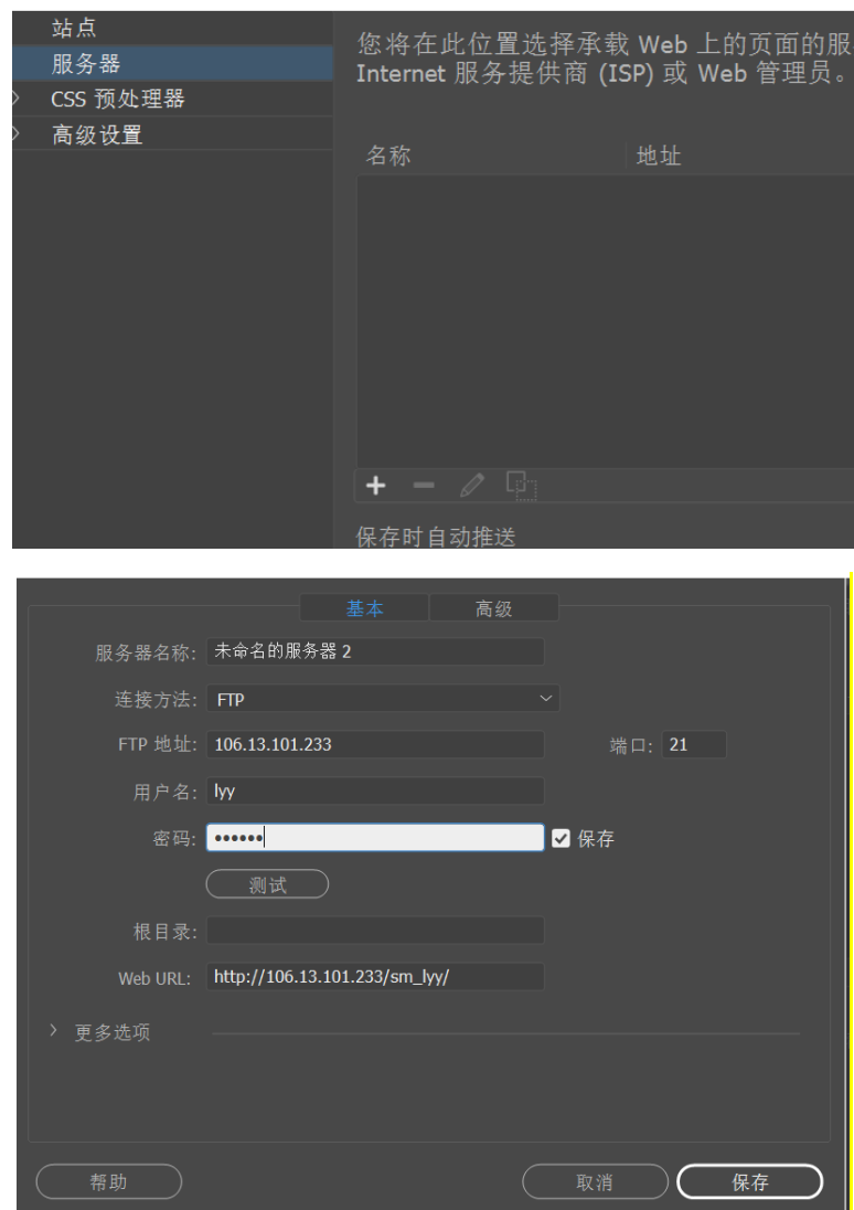
图 5 添加服务器
