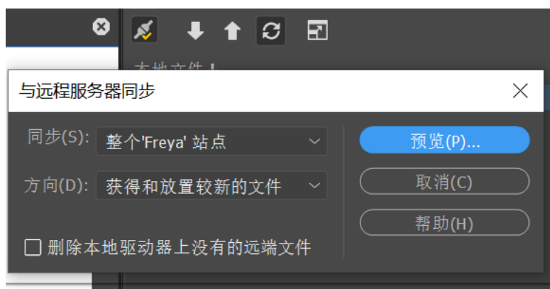
图 8 预览文件
